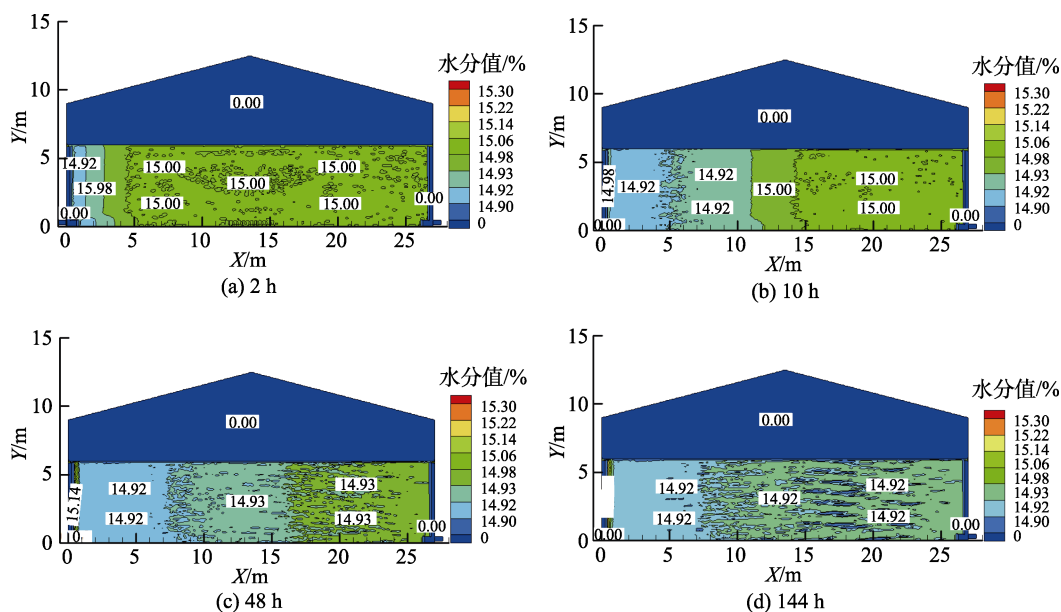
图 6 工况 2 条件下粮堆内部的水分含量分布
