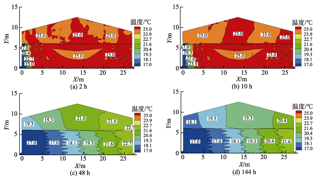
图 2 工况 1 条件下粮堆内部的温度分布
