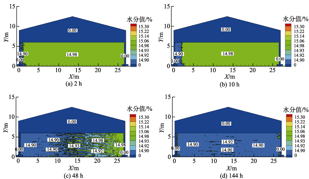
图 7 工况三条件下粮堆内部的水分含量分布
